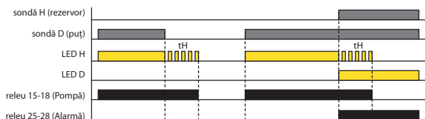
REZERVOARE - REZERVOR, TEMPORIZARE OFF (Funcția 8)
