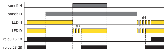
POMPARE GOLIRE, TEMPORIZARE ON (Funcția 6)
