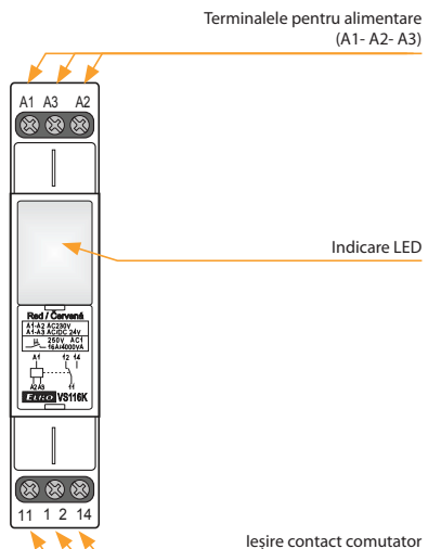
Terminal A3 numai pentru VS116K
