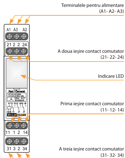
Terminal A3 numai pentru VS308K
