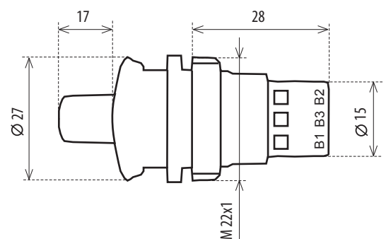
Potențiomtru extern for CRM-2HE, CRM-91HE
