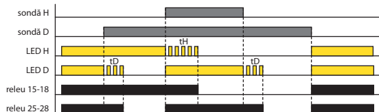
POMPARE GOLIRE, TEMPORIZARE OFF (Funcția 6)
