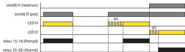
REZERVOARE - REZERVOR, TEMPORIZARE ON (Funcția 8)
