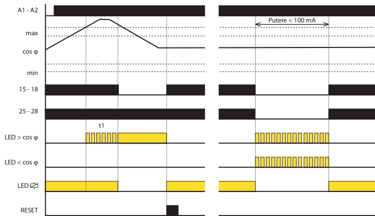
Memorie activată, două moduri releu
