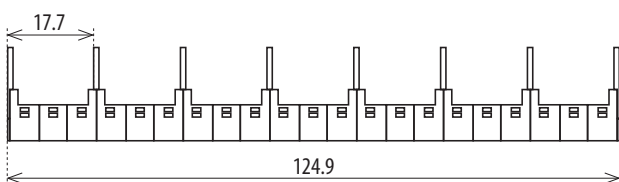
Pas conexiune CB-17-8
