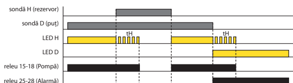
PUȚ - REZERVOR, TEMPORIZARE OFF (Funcția 7)
