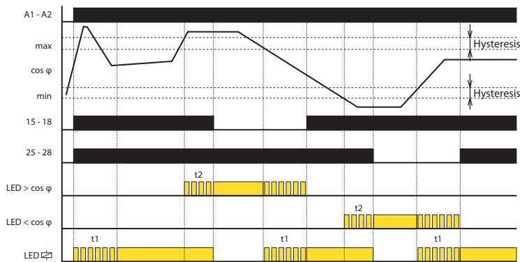
Memorie activată, două moduri releu
