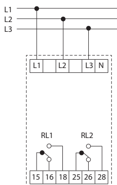
3 - conductori
