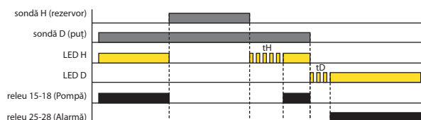
PUȚ - REZERVOR, TEMPORIZARE ON (Funcția 7)
